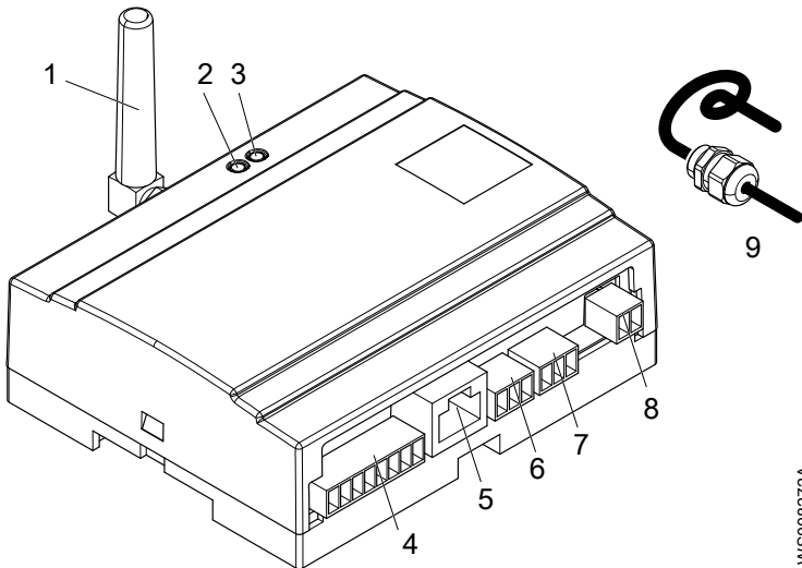
Figur 1: CCD301, reservedelsnummer 803 49 00
