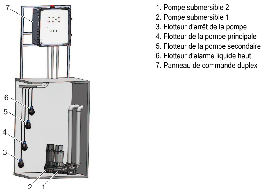
Figure 1: Installation typique du panneau de commande duplex de la série 3DWS/4DWS
