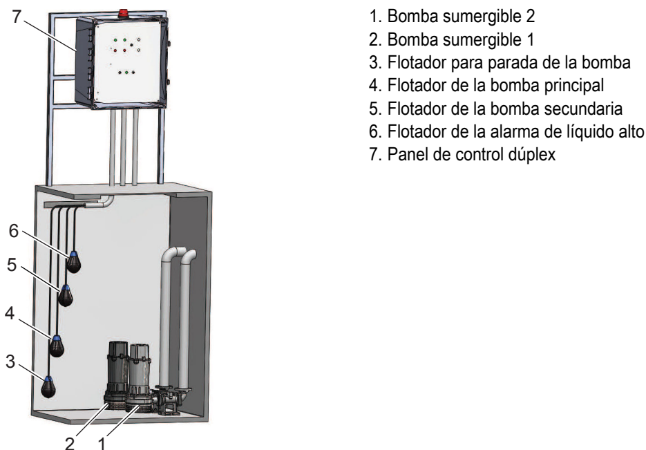
Figura 1: Instalación típica del panel de control dúplex 4DWC
