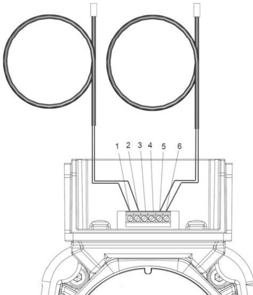
Figure 3: Schéma de raccordement pour ecocirc 20-18+ pour le contrôle de température unique ou de type « delta T ».
