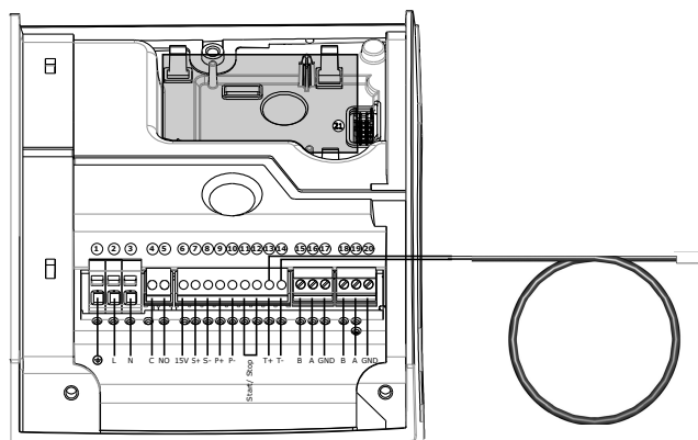
Figure 1: Schéma des raccordements pour les modèles monophasés ecocirc XL
