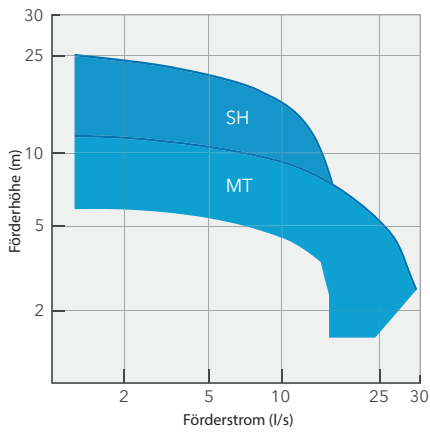
Flygt-Serie 3085
