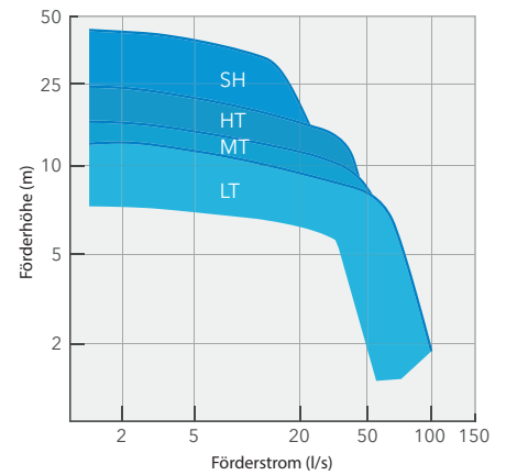
Flygt-Serie 3127
