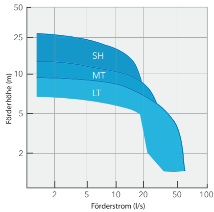
Flygt-Serie 3102
