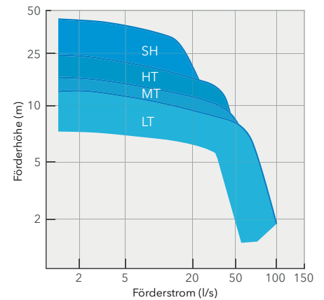
Flygt-Serie 3127
