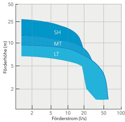
Flygt-Serie 3102
