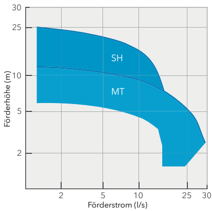
Flygt-Serie 3085
