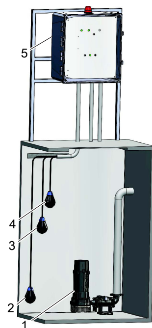
Figura 1: Instalación típica del panel de control simple 3SD/4SD
