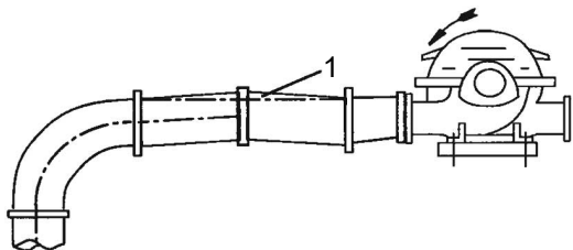
Figura 8: Tubo de aspiración instalado con una elevación gradual hacia la bomba: correcto
