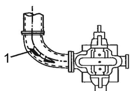
Figura 15: Tubo de aspiración por encima de la bomba: incorrecto
