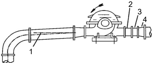
Figura 7: Carga inestable de impulsor de aspiración doble
