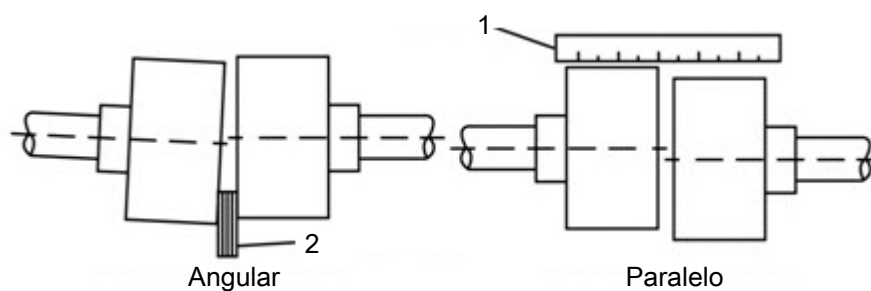
Figura 3: Verifique la alineación utilizando un borde derecho: correcto.
