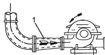
Figura 14: Tubo de aspiración por encima de la bomba: correcto
