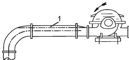
Figura 10: Tubo de aspiración instalado con un reductor: incorrecto
