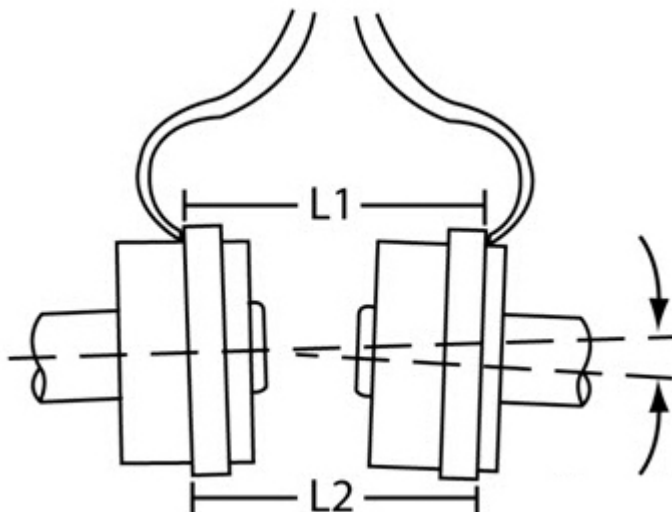
Figura 5: Verifique la alineación usando calibradores
