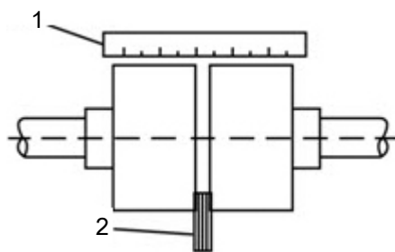
Figura 3: Verifique la alineación utilizando un borde derecho: correcto.
