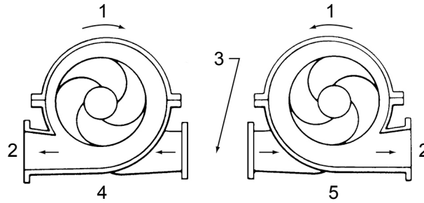
Figura 16: Corrija la relación del impulsor y la carcasa
