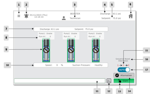
Figura 5.1.1. Pantalla Inicio
