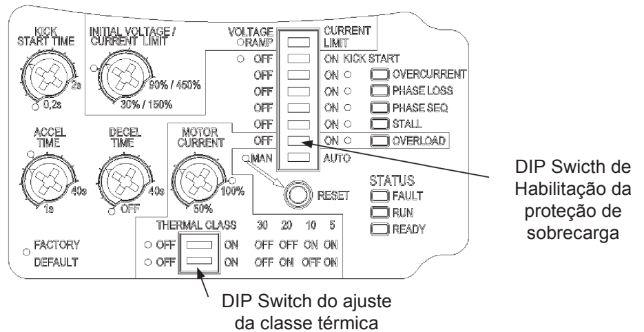
Figura 4.10 - Habilitação e ajuste de proteção de sobrecarga
