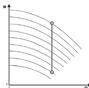
Konstantmengenregelung
