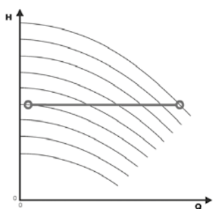
Konstantdruckregelung
