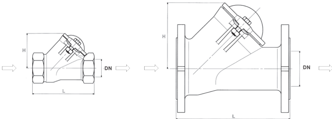
MODELL Rp 1 1/4 - 1 1/2 - 2
