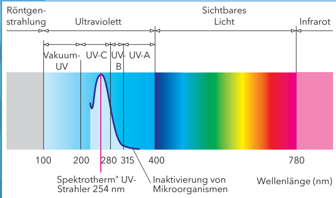
UV ist sehr energiereiches Licht mit einer Wellenlänge von 200-400 nm. Besonders wirksam zur Desinfektion von Wasser ist UV-Licht mit 254 nm.
