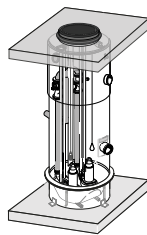
TOP VD för installation i vägytor med trafik last. Med gjutjärnsbetäckning och avlastningsplatta för Klass D last. Prefabricerad förankringsplatta som option.
