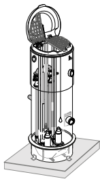
TOP MP för installation i grönytor. Med ventilerat lock av stabil GRP plast. Prefabricerad förankringsplatta som option.
