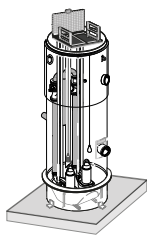
TOP MA för installation i grönytor. Med Abat lucka. Prefabricerad förankringsplatta som option.
