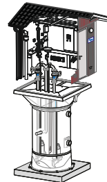
TOP HT med servicebyggnad. Flera storlekar på byggnad. Prefabricerad förankringsplatta som option.
