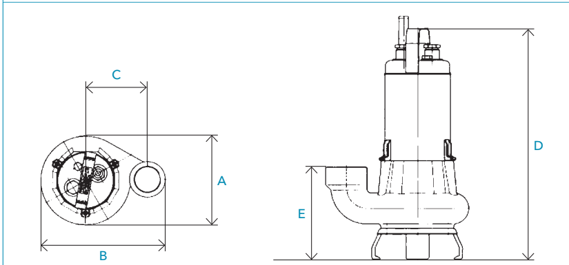
Måttskiss: DL/DLV 50-serien
