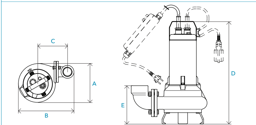
Måttskiss: DL/DLV 50-serien
